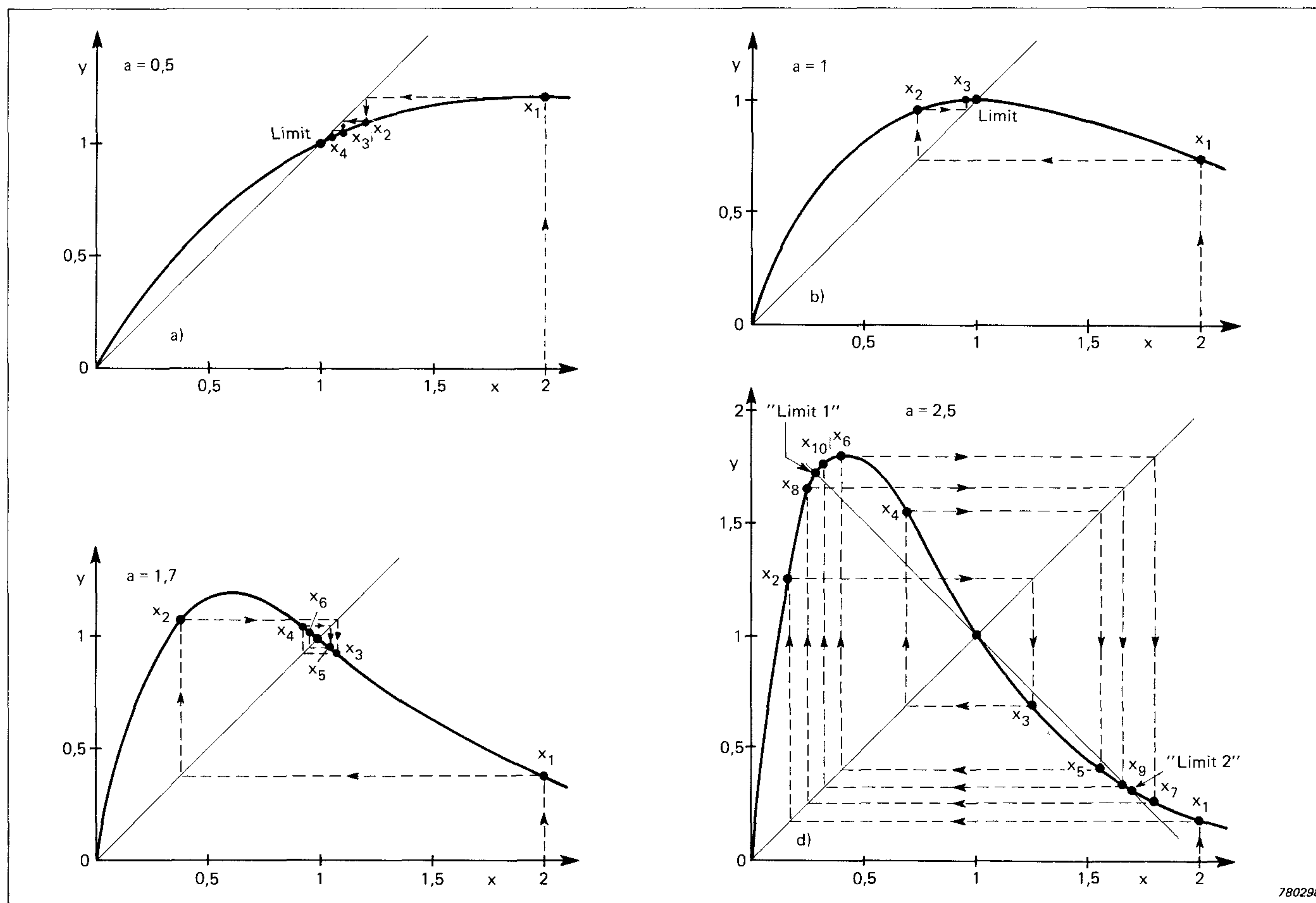
Fig.2. The compressor function for different values of a a) a = 0,5 c) a = 1,7 b) a = 1 d) a = 2,5
